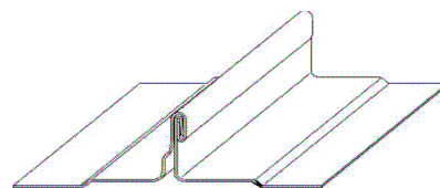
Doppelstehfalz mit Clip Relief
